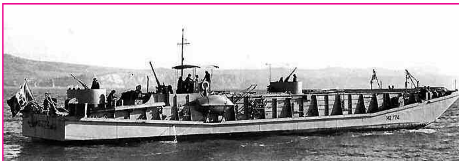
MZ 774 - tipo MZ, seconda serie - Dislocamento: 278 tonnellate - Velocità: 10 nodi - Lunghezza 47 metri - Larghezza 6,5 metri - Equipaggio: 14 - Armamento: 1 pezzo da 76/40, 2 da 20/70 - Nota: unità adatta al trasporto di carri armati; stiva più alta e portellone rinforzato - Da Navi e Relitti tra il promontorio di Portofino e Punta Mesco - di Emilio Carta
